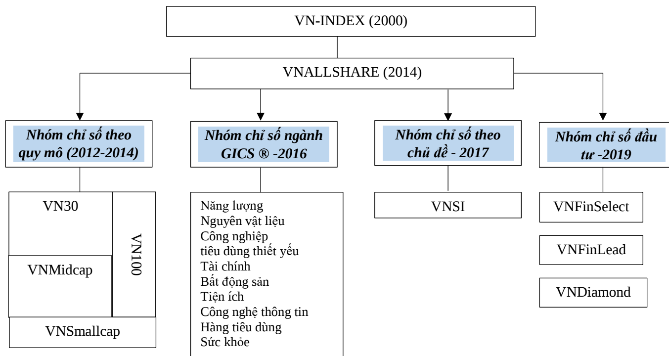
Hình 2: Cấu trúc bộ chỉ số HOSE-Index
